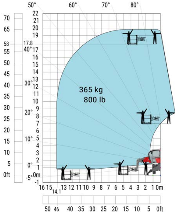
Maszyna na stabilizatorach, z obrotową wieżą, z platformą 365 kg
