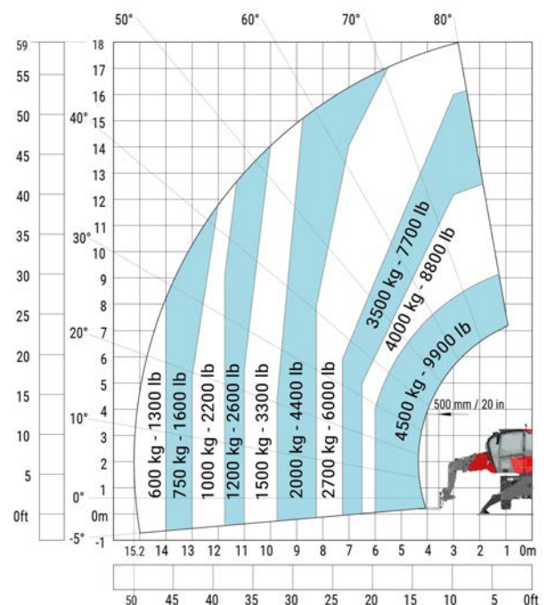
Maszyna na stabilizatorach, z obroconą wieżą, z widełmi
