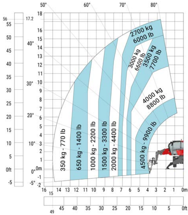
Maszyna na stabilizatorach, z obrotową wieżą, z wciągarką 5000 kg
