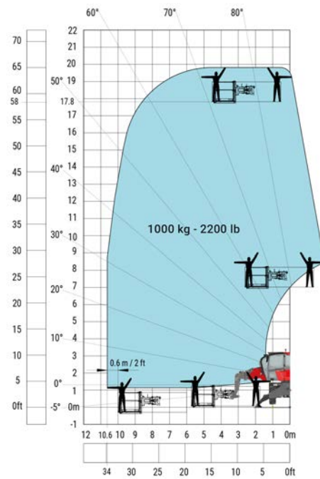
Maszyna na stabilizatorach, z obrotową wieżą, z platformą 1000 kg
