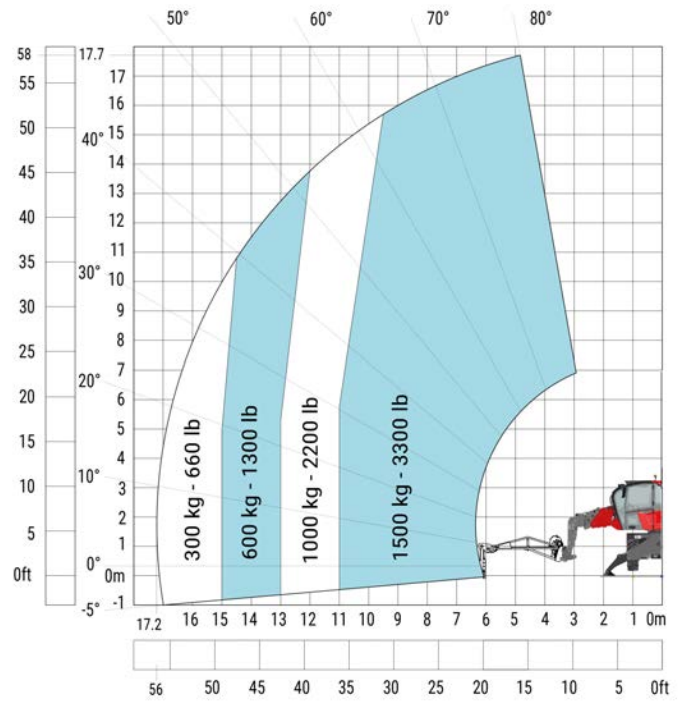
Maszyna na stabilizatorach, z obrotową wieżą, z wysięgnikiem 1500 kg
