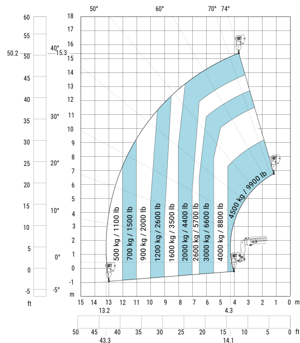
Maszyna na stabilizatorach, z obroconą wieżą, z wciągarką 5000 kg
